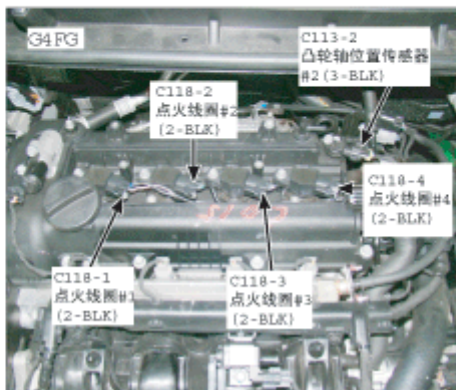
20. 发动机顶部
