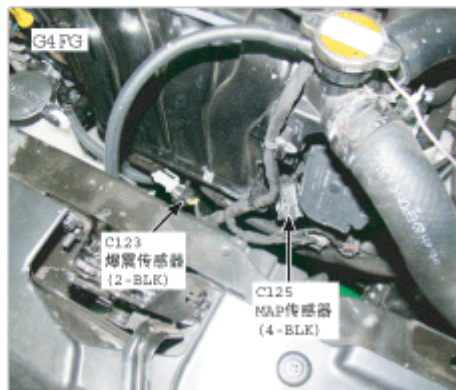
21. 发动机左侧
