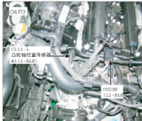
24. 发动机后侧
