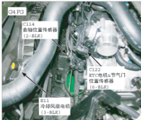
23. 发动机左侧
