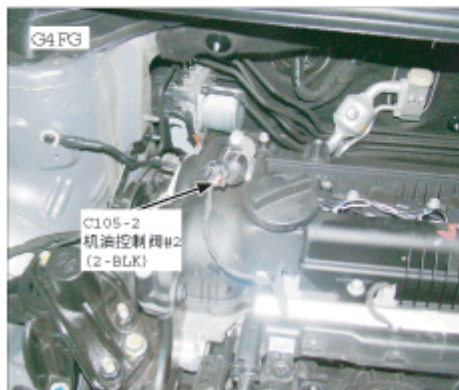
19. 发动机顶部
