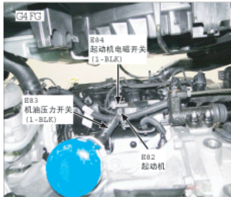
22. 发动机左侧 (底部视图)
